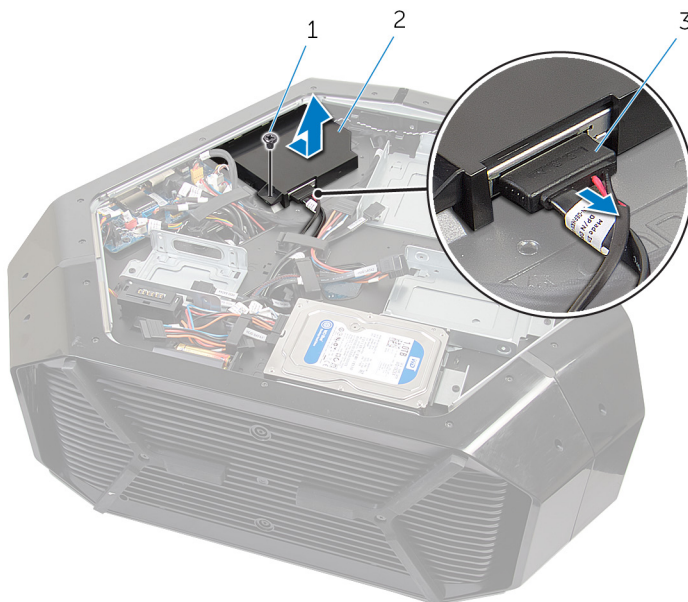
Рисунок 13. Извлечение оптического дисковода в сборе
