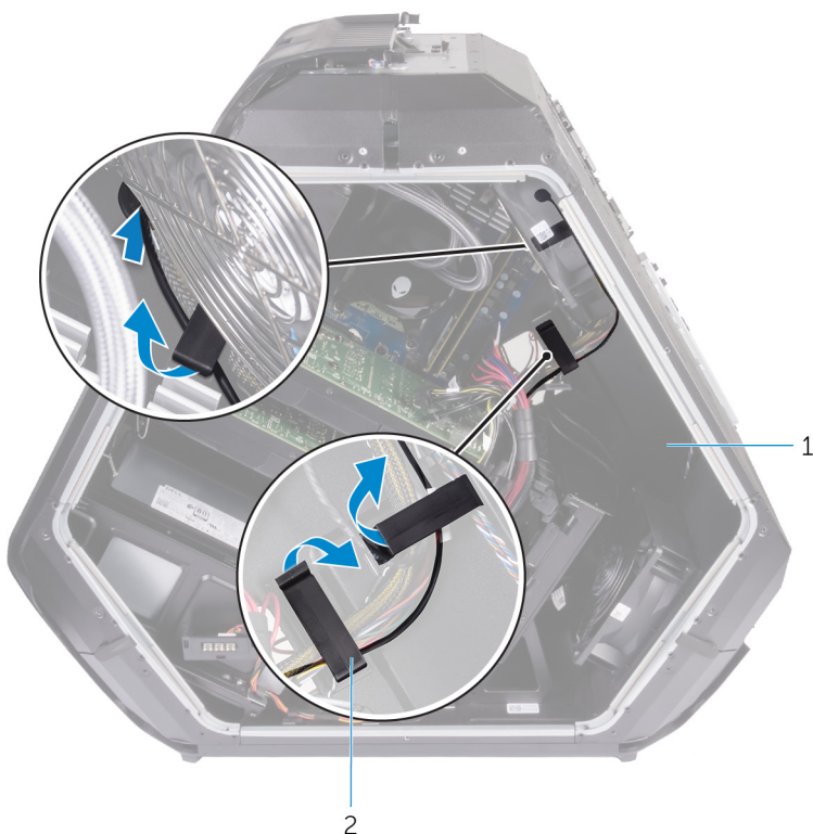
Рисунок 64. Извлечение кабеля платы кнопки извлечения лотка оптического дисковод
