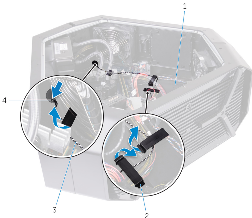
Рисунок 67. Извлечение кабеля подсветки задней панели ввода-вывода
